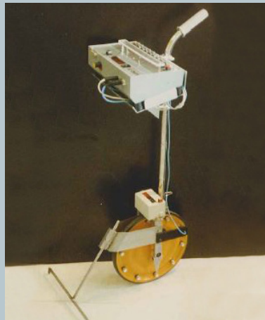
Figure 4 – Le CRR possède une expérience de plusieurs années dans le domaine des inspections visuelles. Ces photos illustrent quelques outils du passé permettant de réaliser rapidement et efficacement une inspection visuelle
