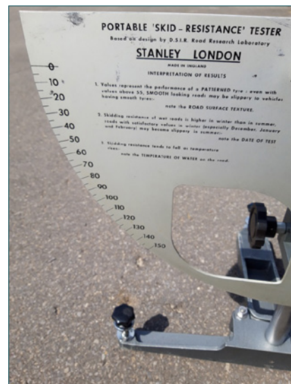
Figuur 4 – Arbitraire schaal van de SRT-slinger (Pendulum Test Value, PTV)
