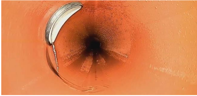
Foto 68 (Bron BRRC) Inlaat met zadelhulpstuk BCA-B
