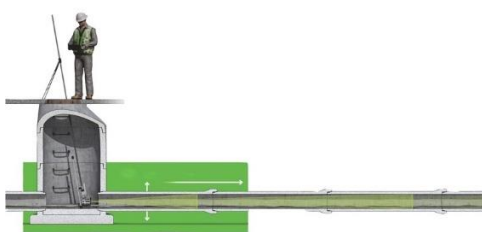
Foto 65 (Bron EnviroSight) Grafische voorstelling - EnviroSight
