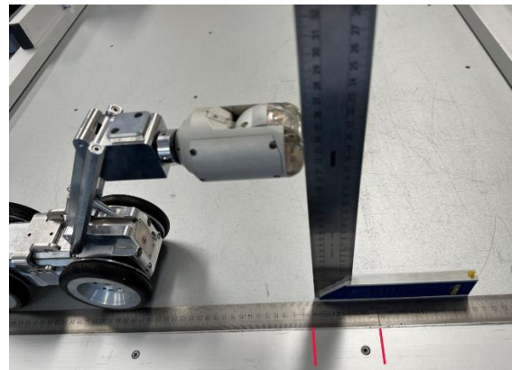
Foto 93 Maximale pantograaf (lift) (Bron BRRC)
