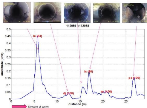
Foto 53 (Bron C4Sewer) Sewerbatt Grafiek met corresponderende foto's
