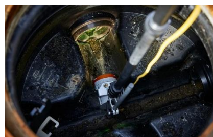
Foto 67 (Bron IBAK) Zoomcamera ASPECTA
