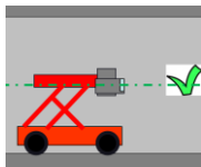
Foto 63 (Bron BRRC) cameralens correct gepositioneerd. In neutrale stand verschijnt de voeg onder en boven gecentreerd in beeld.
